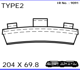
PL70072 THK 48.4
