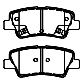
PL25337 THK 15.6
