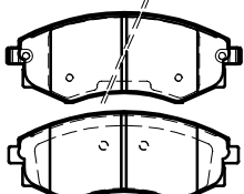
PL80105 THK 17
