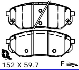
PL21553 THK 14
