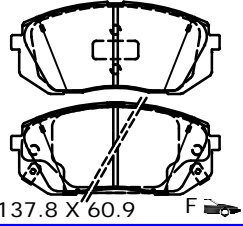
PL24317 THK 17.5
