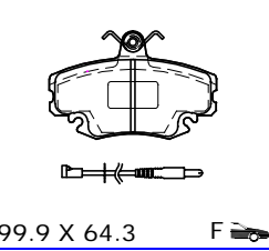
PL21463 THK 18.2
