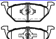
PL23130 THK 19.2
