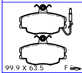
PL21979 THK 18
