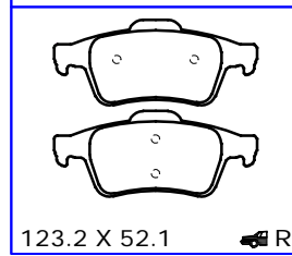
PL24137 THK 16.7
