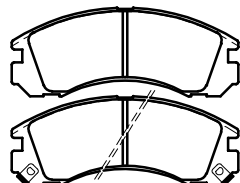
PL21370 THK 15.7
