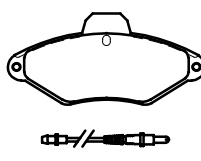
PL21631 THK 17
