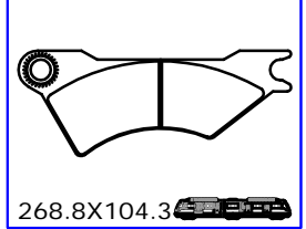
PL70047 THK 17
