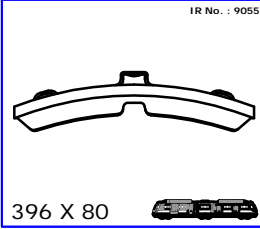
PL70073 THK 45.8
