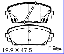
PL25365 THK 16.6
