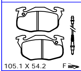
PL21463 THK 18.2
