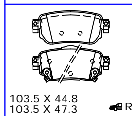
PL25965 THK 15.1
