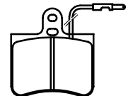
PL20288 THK 16
