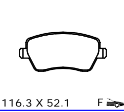
PL23973 THK 17.3
