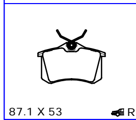
PL23215 THK 18.3
